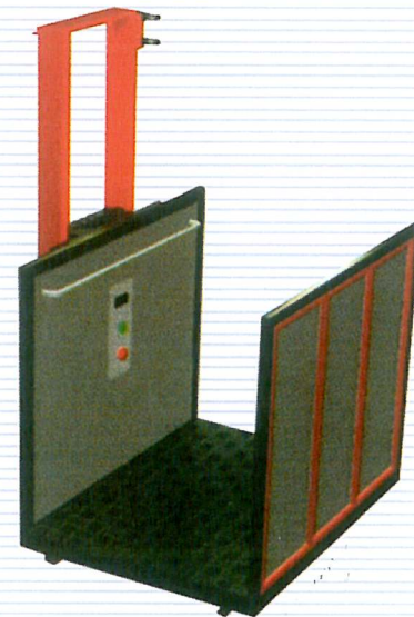
بالابر ویلچر بر هیدرولیک با تجهیزات ایمنی، کلید فرمان
